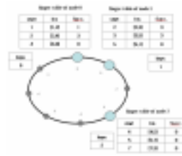
(d) DHT-based P2P
