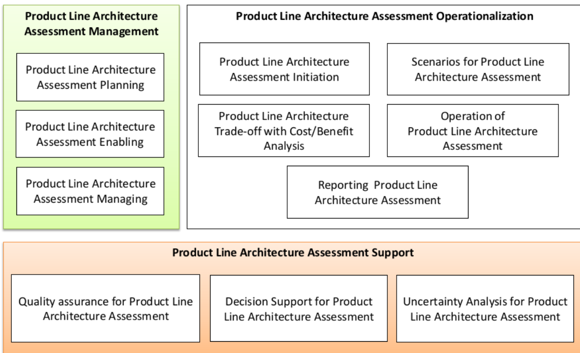
[그림 2] SSPL 아키텍처 평가 핵심 프로세스
