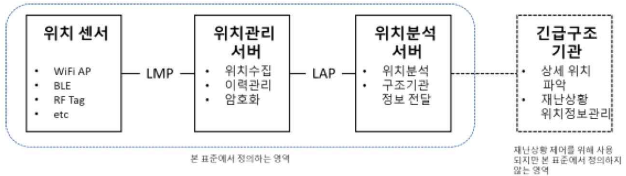
[그림 2] 재난 피해자 위치분석 시스템 구조 다이어그램
