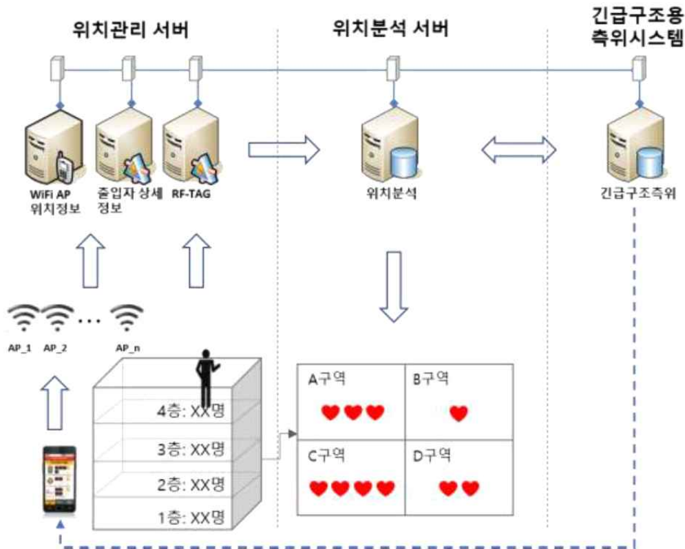
[그림 1] 재난 피해자 위치분석 시스템 개념도
