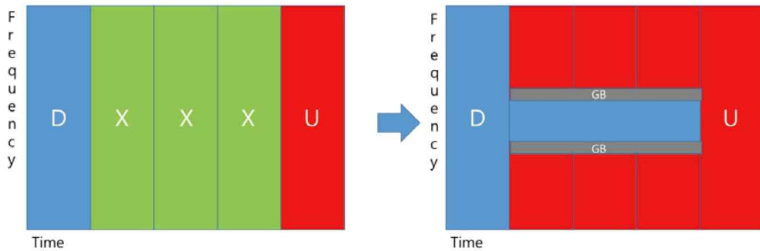
[그림 2] 상향링크 심볼 내에서의 하향링크 허용 방안
