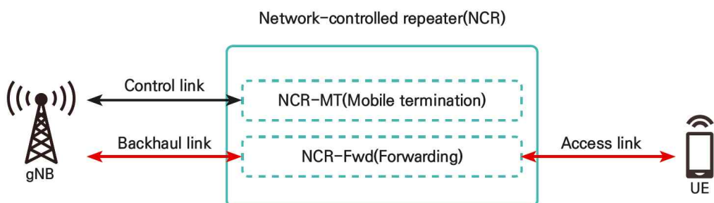
[ 그림 3] Network-Controlled Repeater (NCR)
