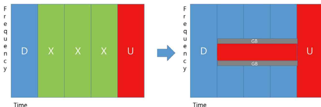
[그림 1] 하향링크 심볼 내에서의 상향링크 허용 방안
