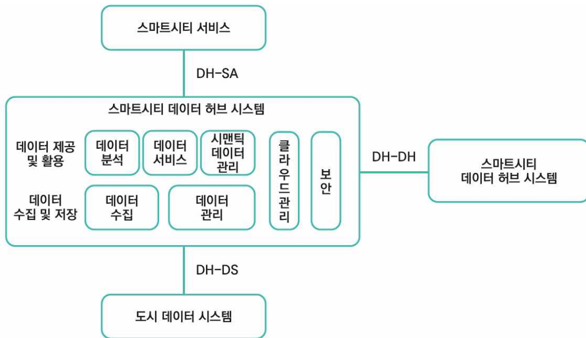
[그림 3] 스마트시티 데이터허브 시스템 참조구조
